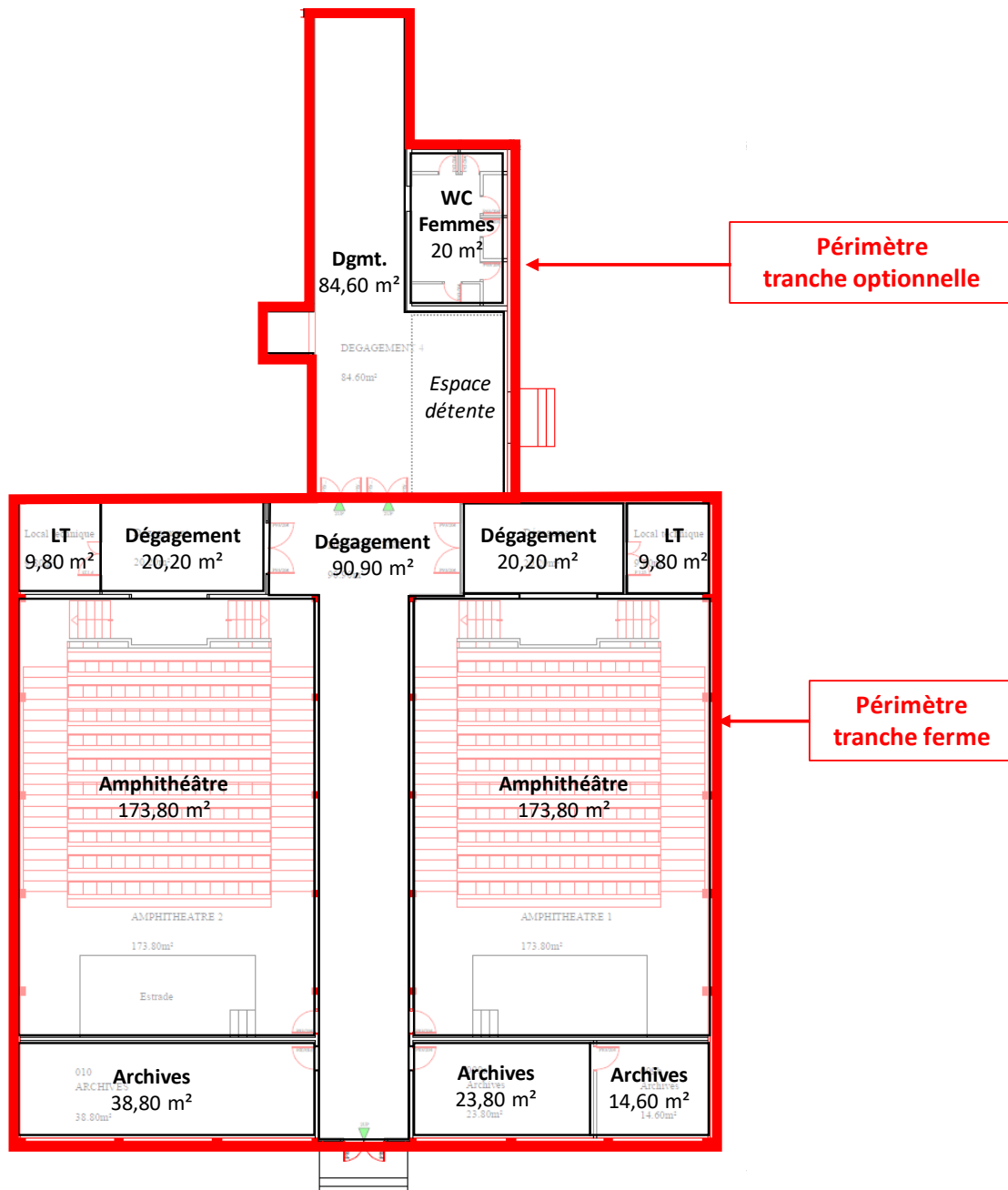
Plan du bloc B du bâtiment F
