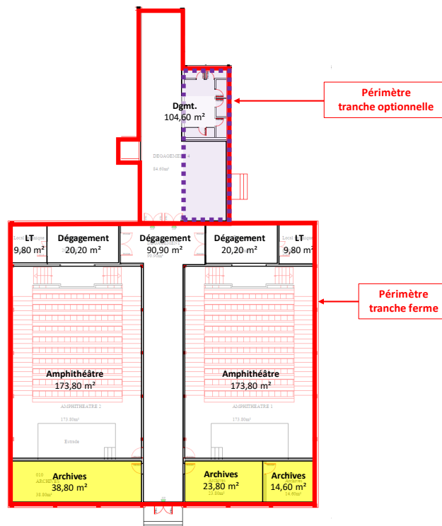
Scénario de faisabilité pour la réhabilitation du bloc B
